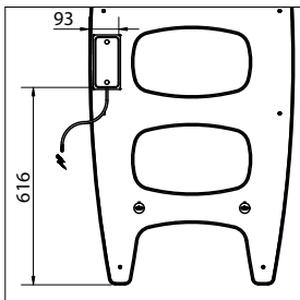
Detail control unit en positie snoer
