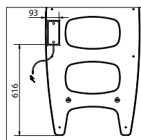
Detail control unit en positie snoer
