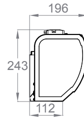
zij aanzicht
