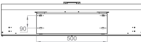
achterzijde
