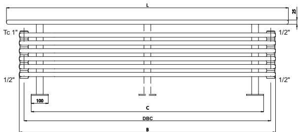
vooraanzicht
