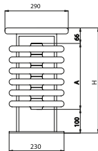
zijaanzicht
