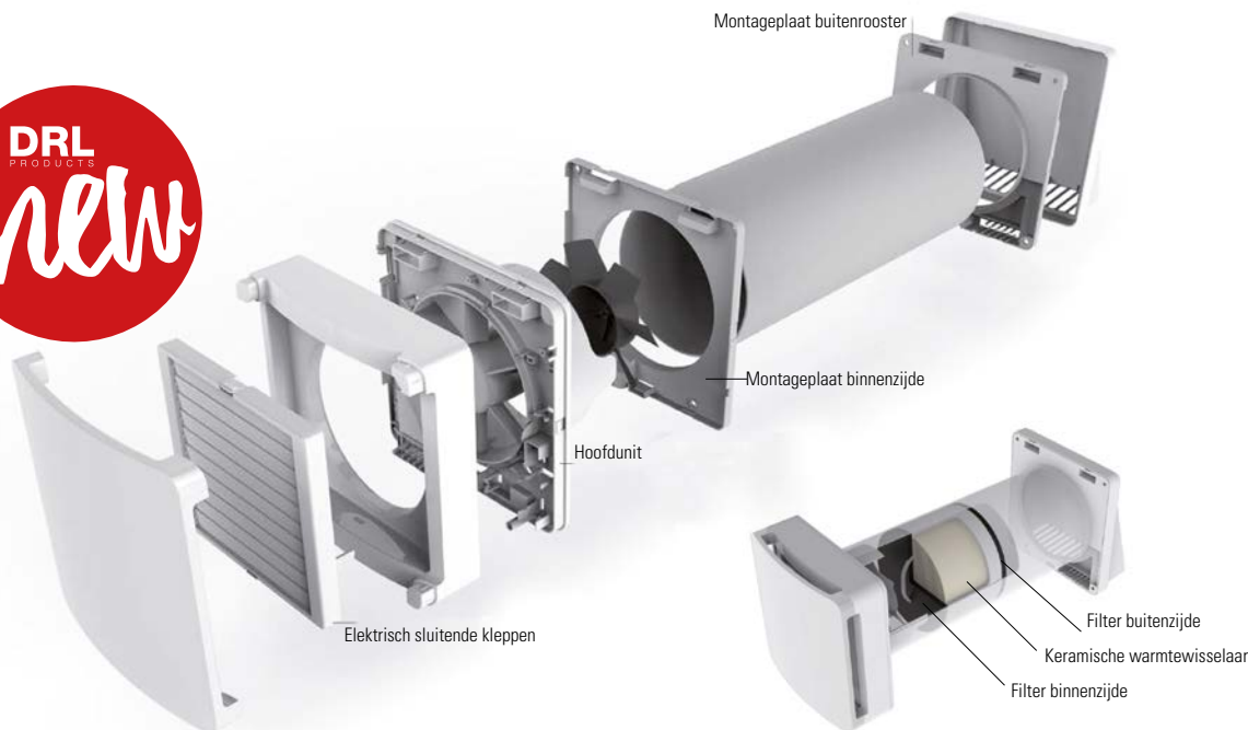
Montageplaat buitenrooster
